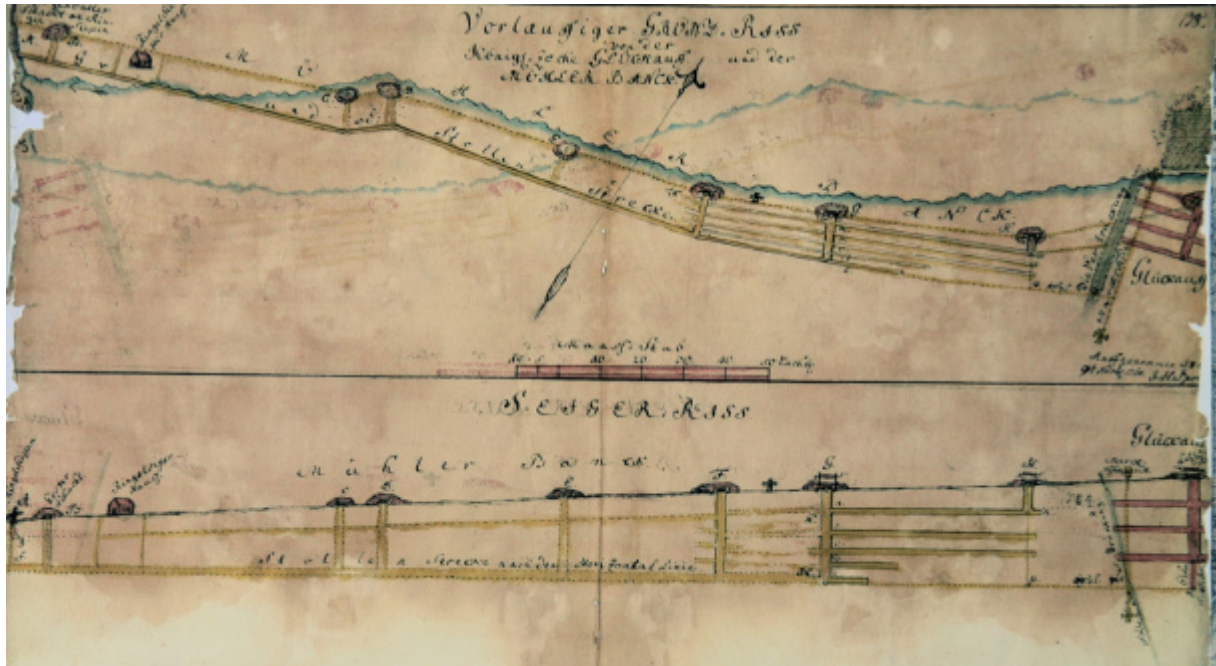
Ältestes bekanntes Grubenbild der Zeche Sieper &Mühler. Oben der Grundriß, unten der Seigerriß (die senkrechte Projektion). Links das Haus ist im Track die Nagelschmiede, ganz rechts der Schacht Amalie von Glückauf. Der Maßstab wird in Lachtern (1 Lachter = 2,08m) angegeben. Im Track zwischen Nagelschmiede und Schacht Amalie.
